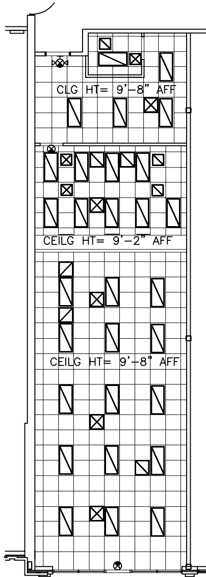
2 REF CLG PLAN SCALE: 1/8"=1'-0"
